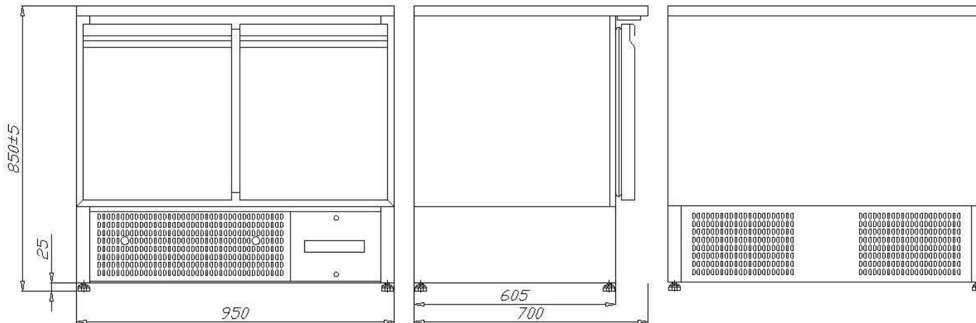
WIDOK OD STRONY OBSŁUGI
